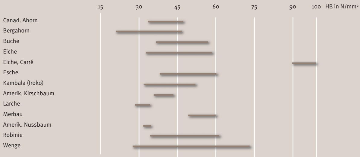
Brinellhärte-Bereiche verschiedener Parkett-Holzarten (bei u = 6 %)
